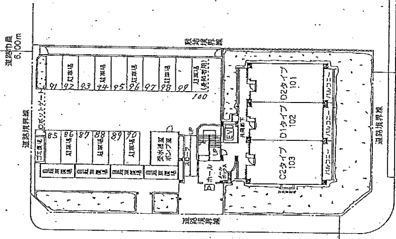
1階平面図
